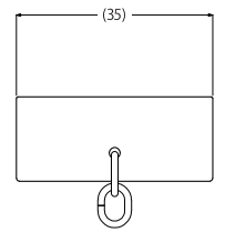
レールキャップ側面図
