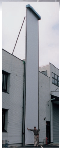
ERF-B200 暗幕仕様 (W2.5m×H15.5m)
